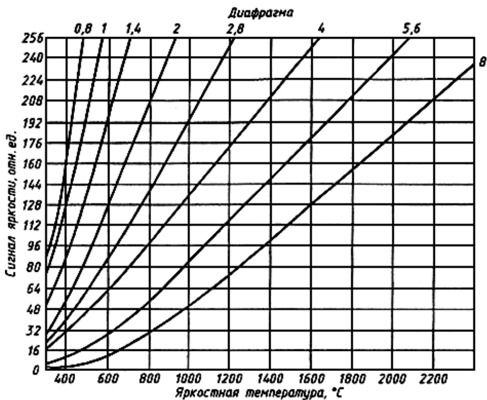
Рисунок Б.1 - Градуировочный график пировидиконной камеры с фильтром N 1
