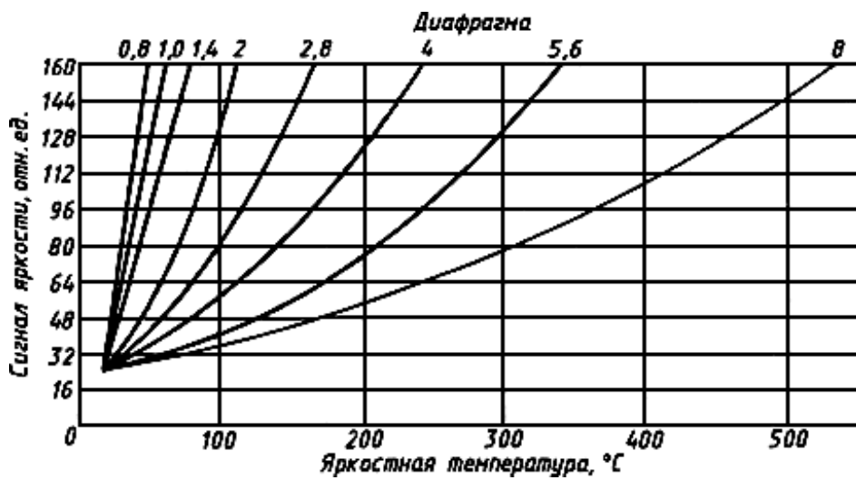
Рисунок Б.2 - Градуировочный график пировидиконной камеры с фильтром N 2
